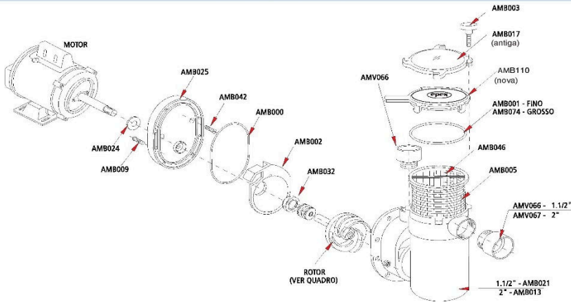
Desenho explodido da bomba
